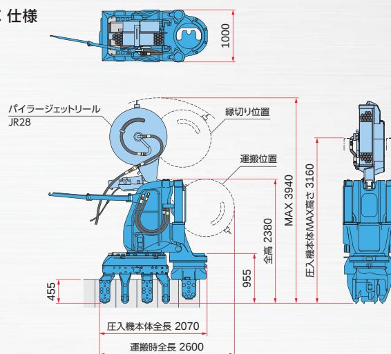
圧入機本体 SILENT PILER F101
